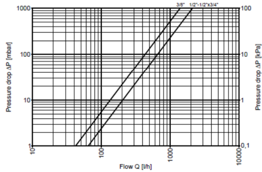
serie 104/1-03-04-045
