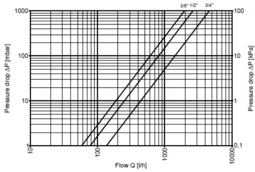
serie 100/1-03-04-05
