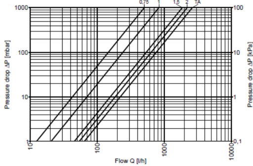
serie 101/1-03
