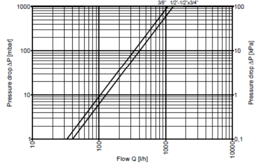
serie 106/1-03-04-045
