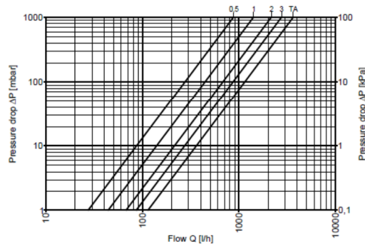
serie 101/1-05
